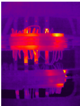
Armário elétrico
