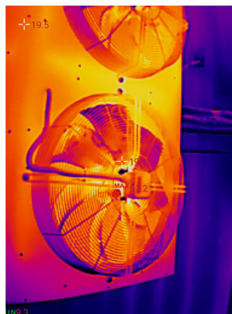
Ventoinha
