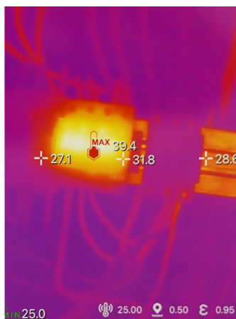
Interruptores elétricos
